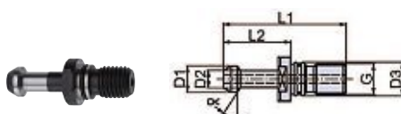
Штревели AZB MAS/VT 30° (JIS B 6339) с внутренним отверстием
