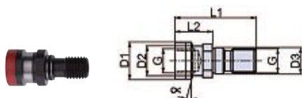
Штревели AZB DIN 2080 с внутренней резьбой
