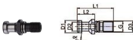
Штревели AZB DIN 69872-B без внутреннего отверстия
