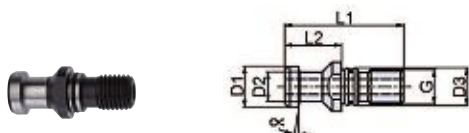
Штревели AZB DIN 69872-A с внутренним отверстием
