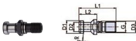
Штревели AZB ISO 7388/II-B с внутренним отверстием
