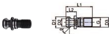
Штревели AZB ISO 7388-B без внутреннего отверстия
