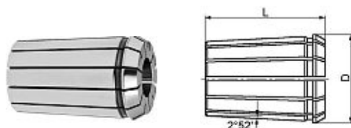
Прецизионные цанги GOZ-DG (двойные шлицы) – 6 мкм или соответственно 10 мкм
