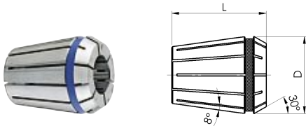
Прецизионные цапги GER-HP – 2 мкм для GER11-HP до GER40-HP
