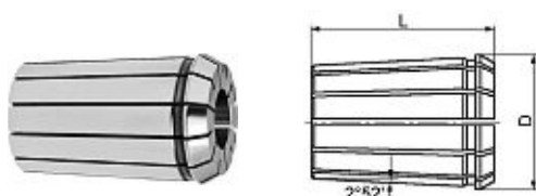
Прецизионные цанги GOZ-DG-HP (двойные шлицы) – 3 мкм
