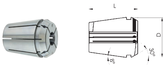
Прецизионные цанги GER-D с внутренним уплотнением для ИК – 5 μm
