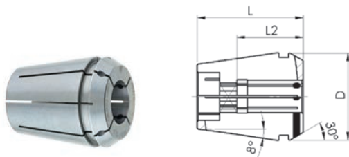
Цанги для метчиков GER-GBD с внутренним квадратом и уплотнением для ИК – 10 μm
