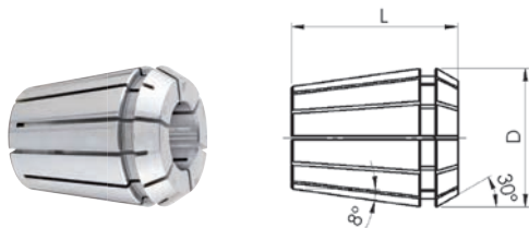
Прецизионные цанги GER-B – 5 μm
